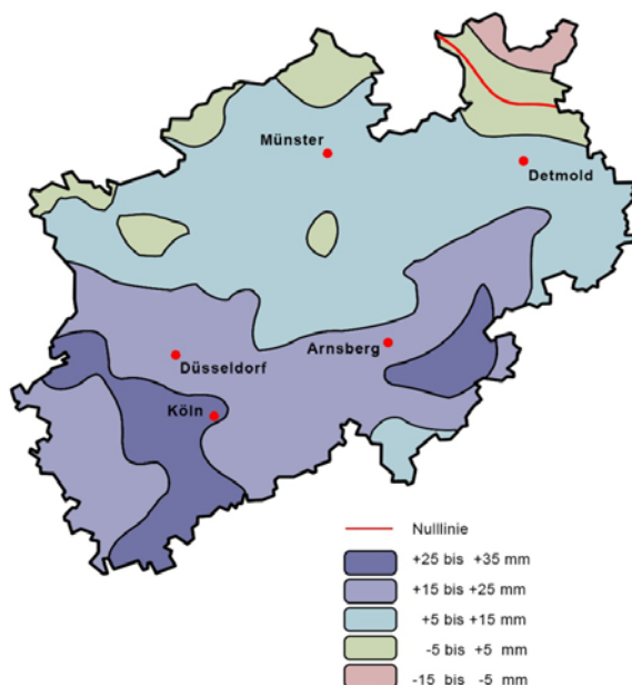
Abbildung 1: Höhenwertänderungen NHN-Höhen im DHHN2016 zu NHN-Höhen im DHHN92
